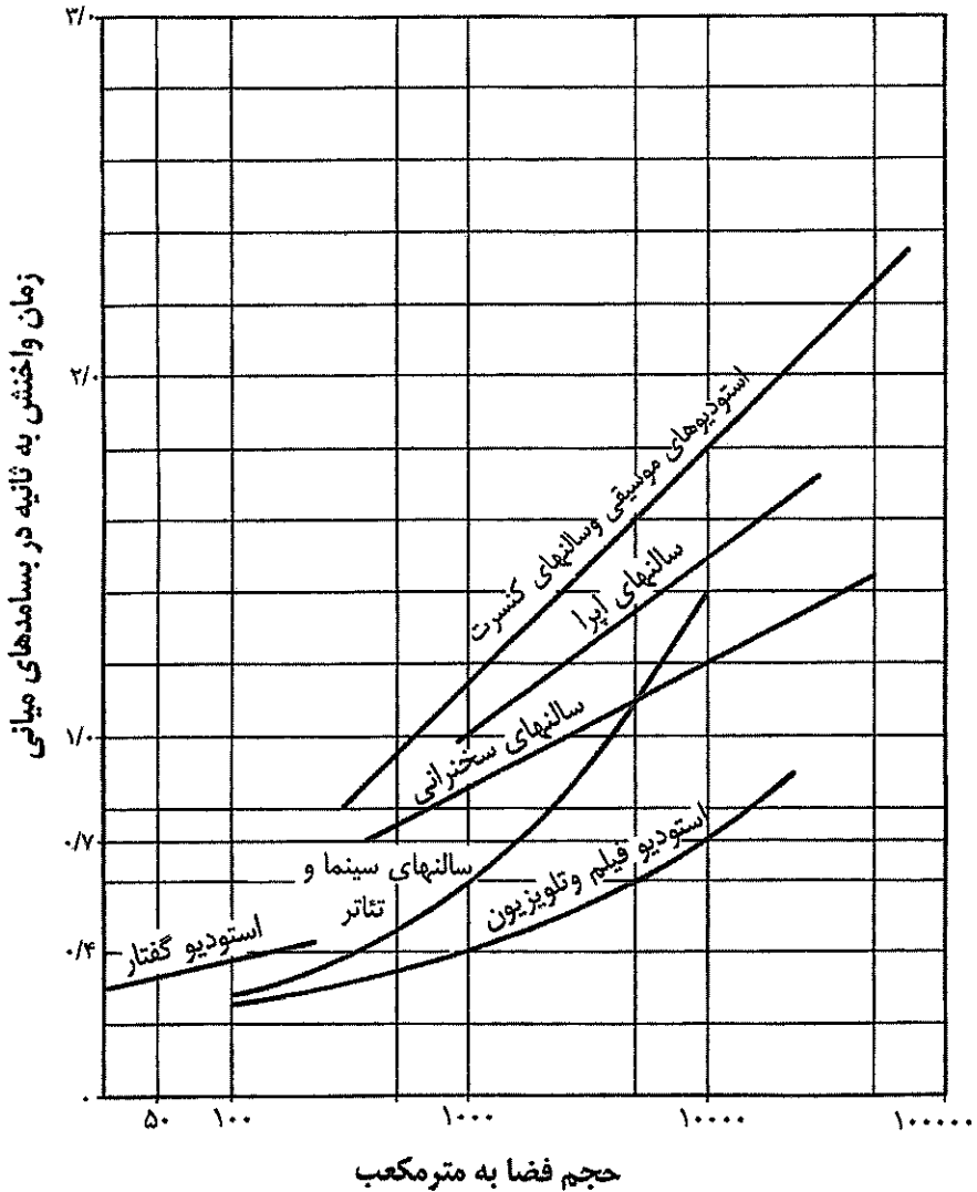
شکل ۱۸-۲-۱: نمودار زمان واخشن بهینه در فضاهای مختلف
